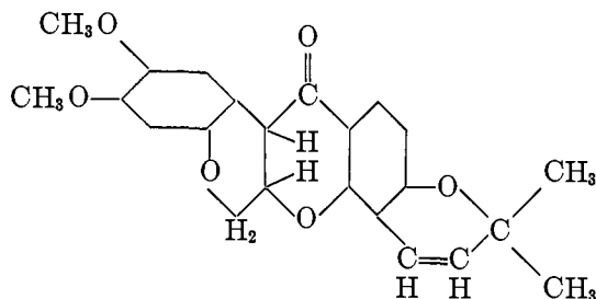
XII
